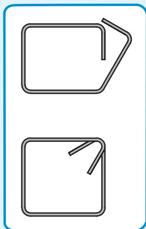
شکل ۴۹-۳- خاموت
