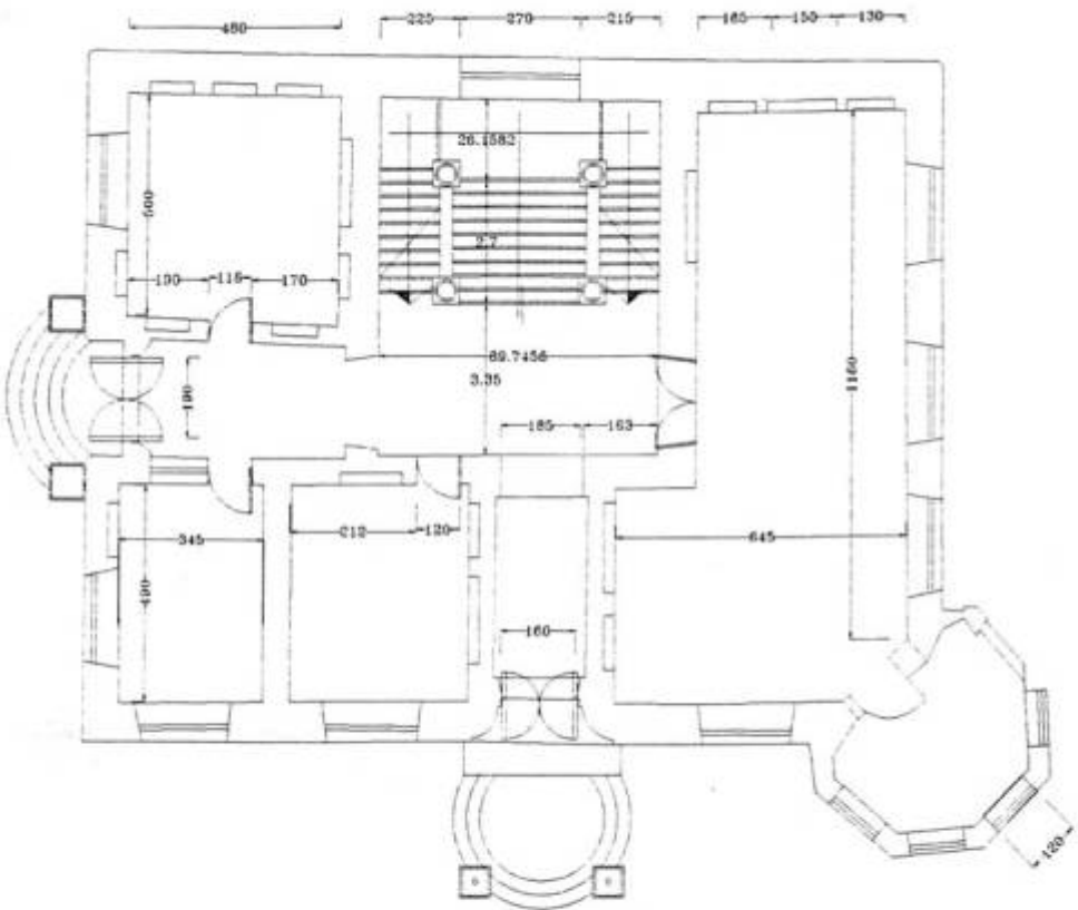
پلان طبقه همکف
