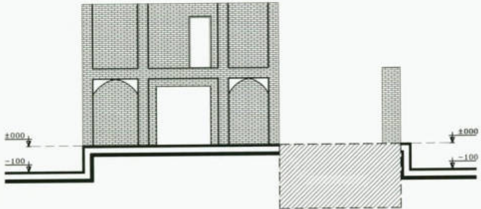
نمای شرقی
