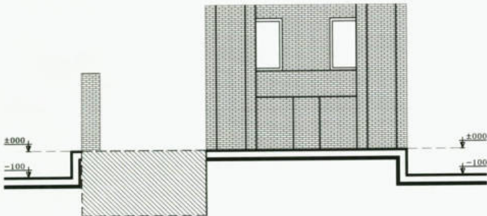
نمای غربی
