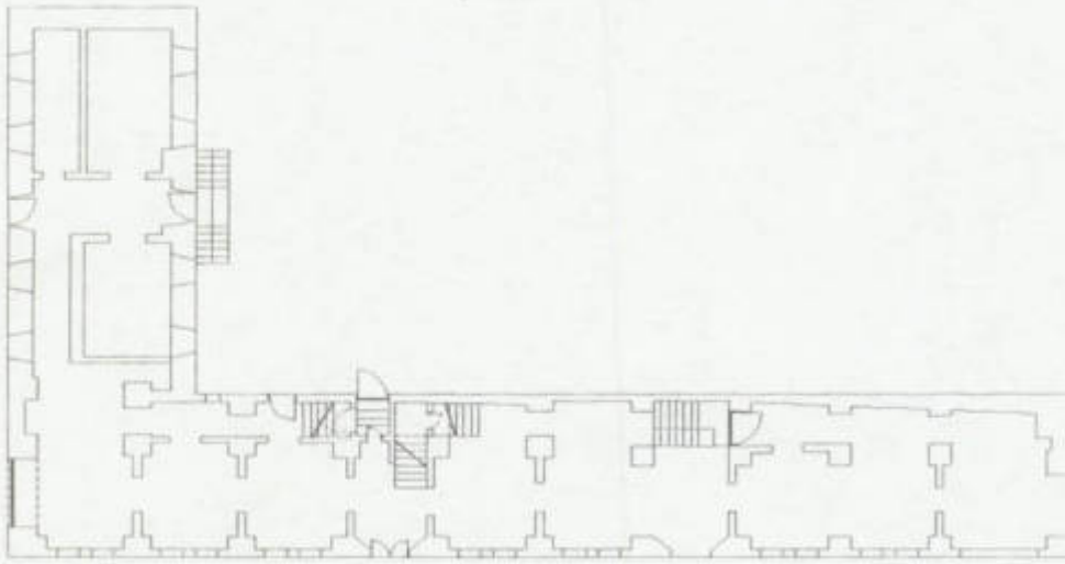
پلان طبقه دوم دانشکده کشاورزی
