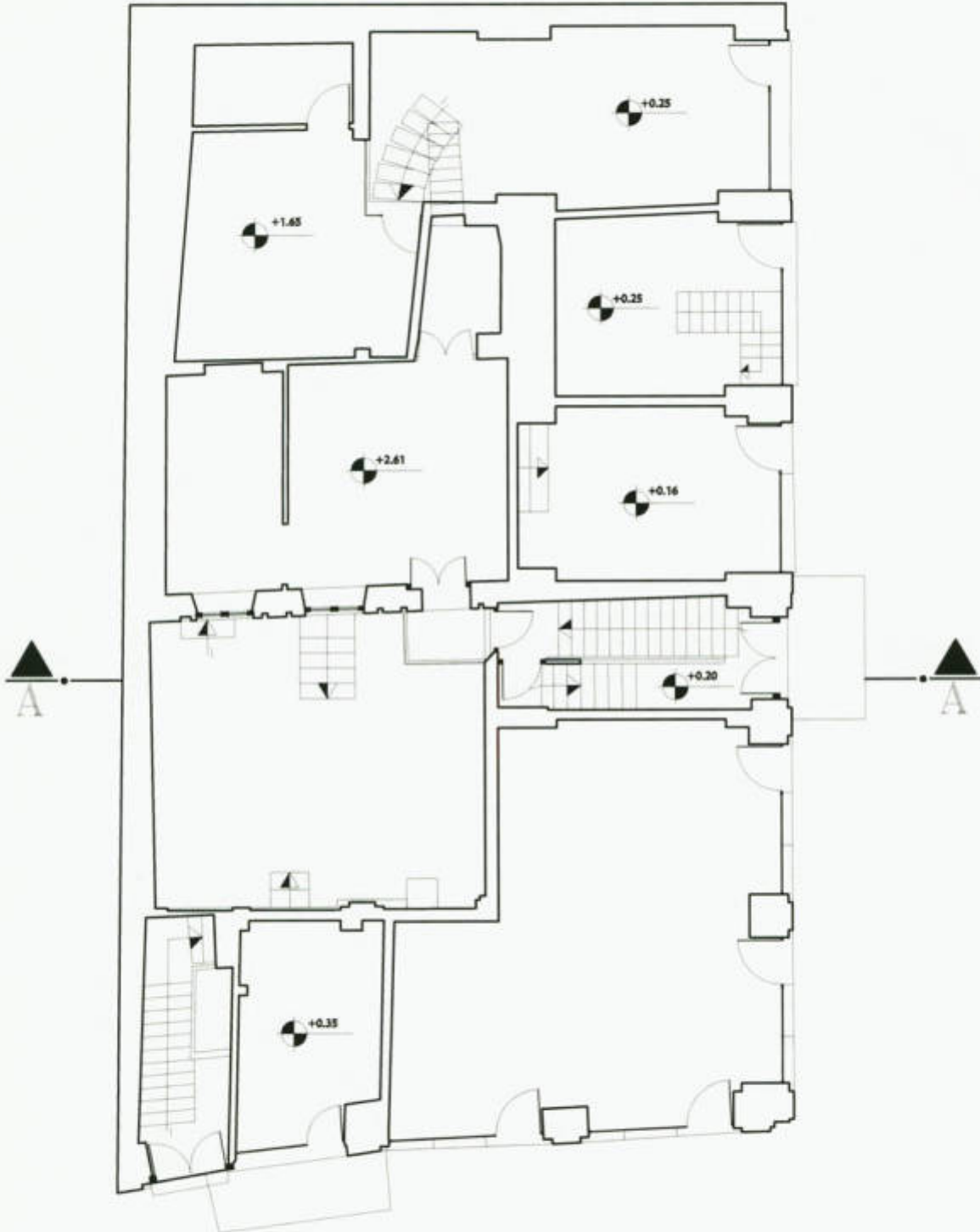
پلان طبقه همکف
