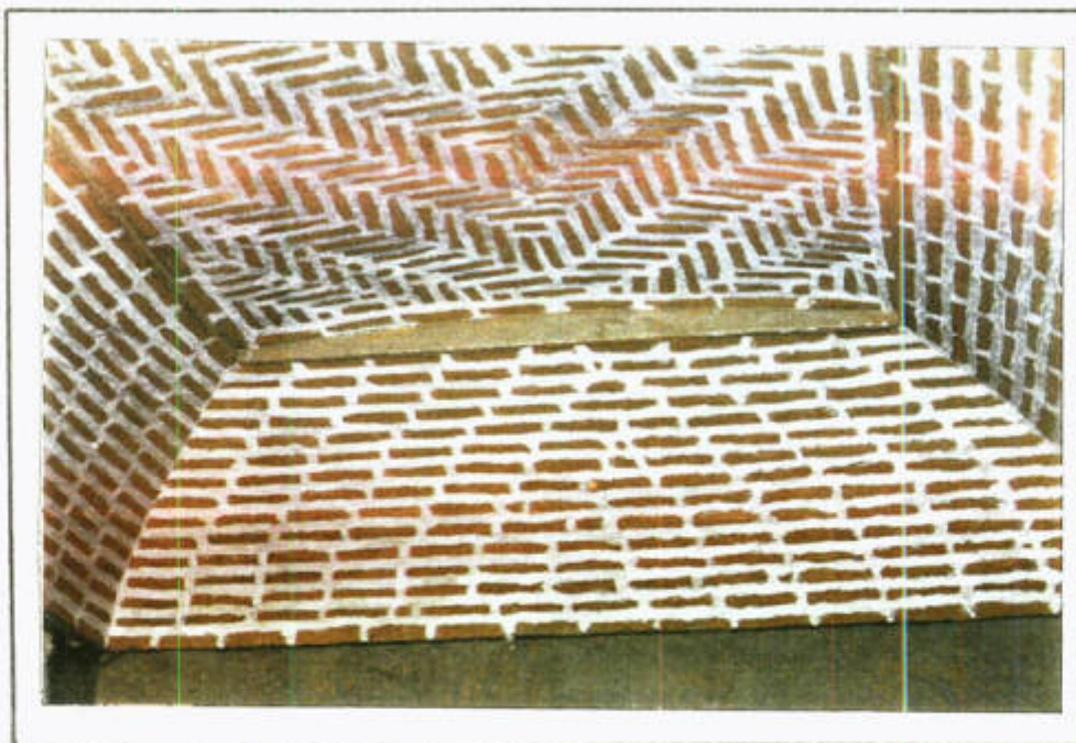
نمایی از مرمت و دوباره سازی طاق آذری در یکی از اتاقهای زیرزمین
