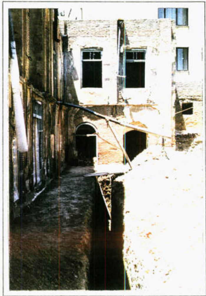
حفر کانال نم زدائی به عمق متوسط ۲۴۰ سانتیمتر
