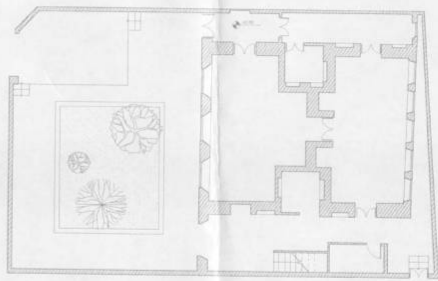
پلان طبقه همکف خانه سیلابی
