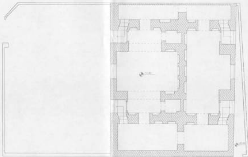
پلان طبقه زیرزمین خانه سیلابی
