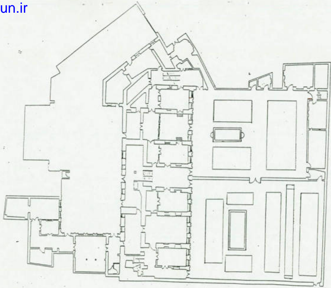
پلان طبقه همکف - خانه امین‌زاده
