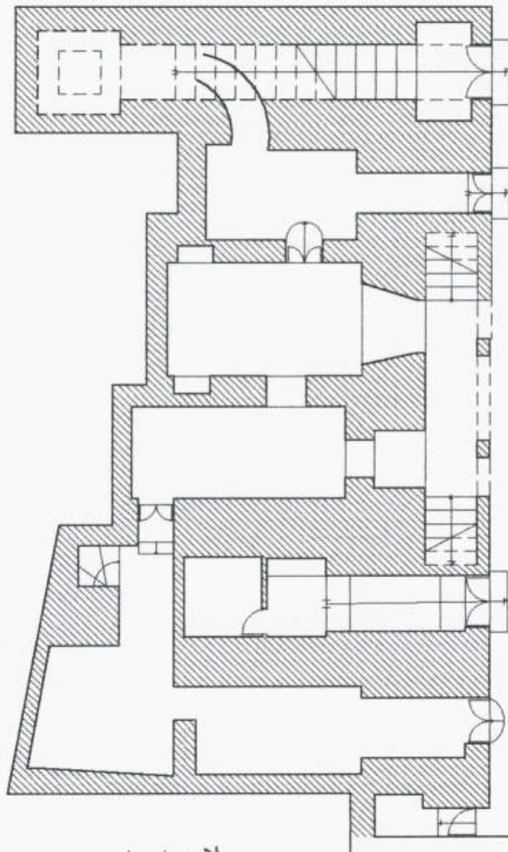
پلان زیرزمین
