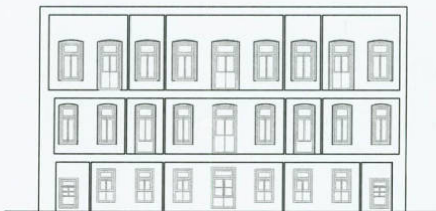
برش A-A
