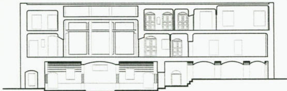
برش الف الف
